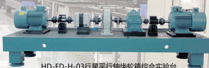
HD-FD-H-03行星平行轴齿轮箱综合实验台
